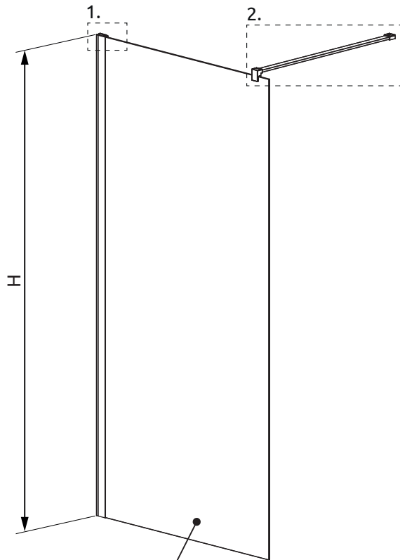
Bild zeigt Einbausituation links
