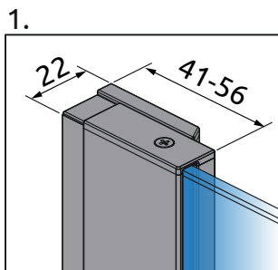
Bild zeigt Einbausituation links
